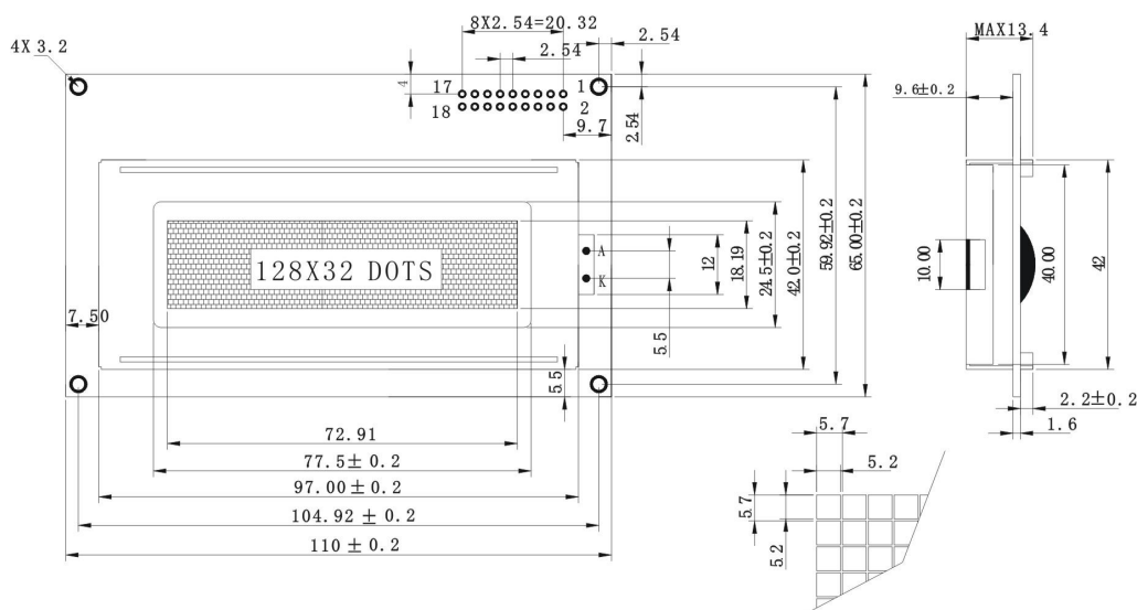
图 1：OCMJ2X8A 模块尺寸图
